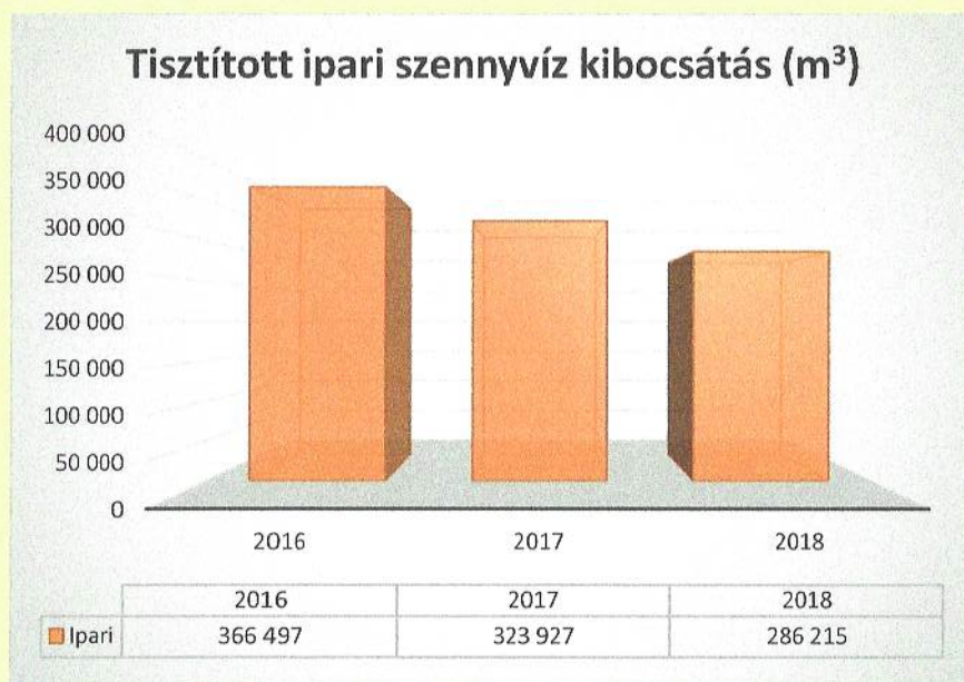
2. diagram - Tisztított ipari szennyvíz mennyiségek
