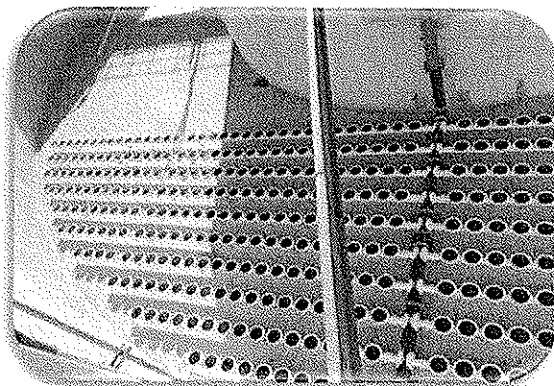
Lezárult a szennyvíztisztító telep felújításának II. üteme. A levegőztető medence építészeti felújítása során a fenék és oldalfalak vízzáró, korrózióálló réteget kaptak. A gépészeti felújítás során a mély-levegőztető rendszer kollektor vezeték és membránfejek (1.314 db) cseréje, banánkeverők és tartószerkezetének cseréje, valamint a szondák cserje történt meg.
